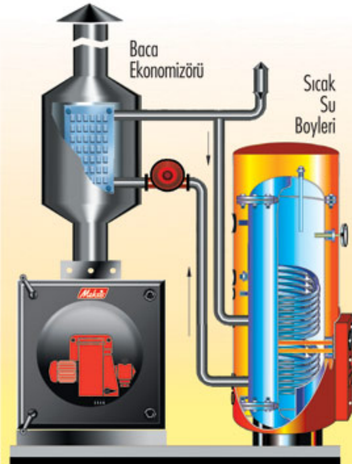
Cimri Plaka "Ekonomizör" Uygulaması
