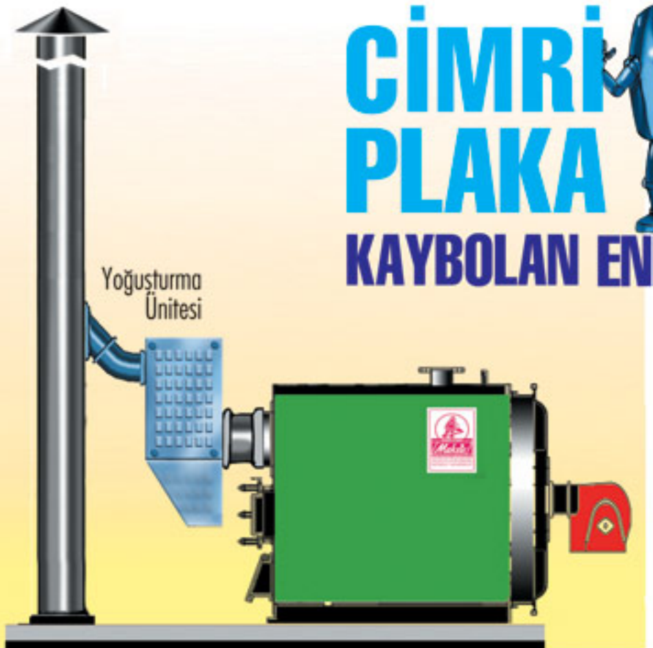
Cimri Plaka "Kondenzasyon Kazanı" Uygulaması
