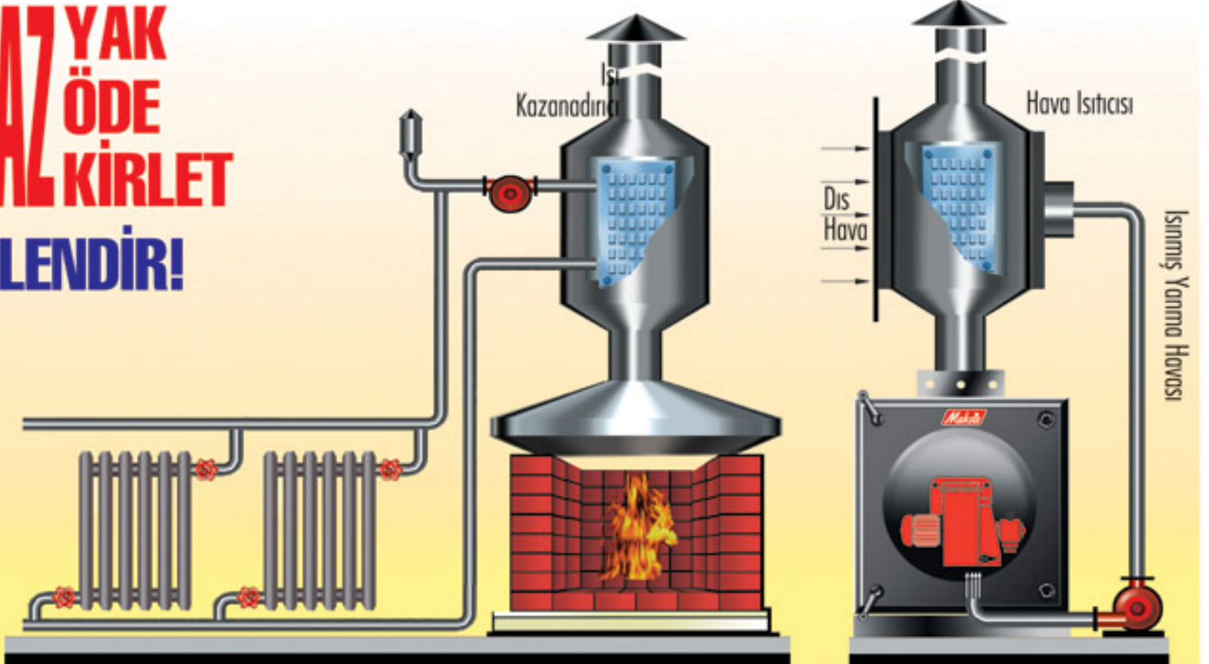
Cimri Plaka "Kazan - Hava Isıtıcı" Uygulaması
