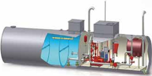
Pompa İstasyonlu Yeraltı Yangın Tankı
