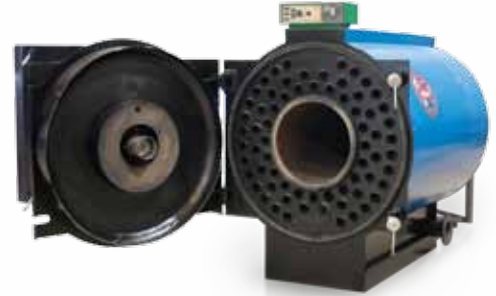
Sıvı / Gaz Yakıtlı Kondenzasyonlu Kazanlar
