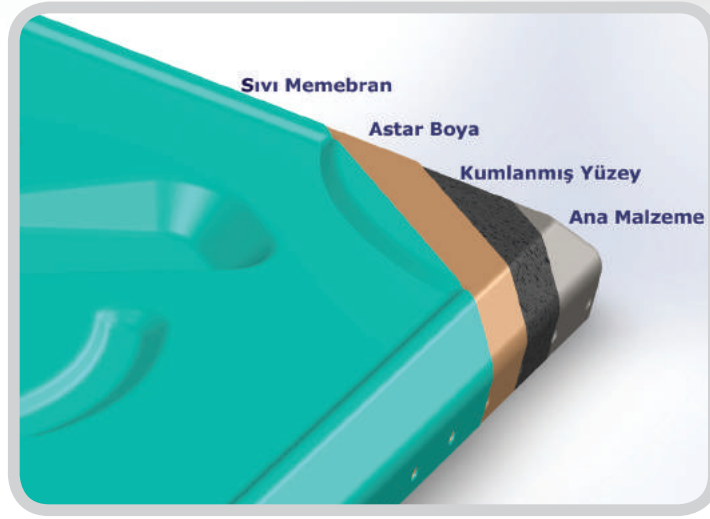
Sıvı Membran Kaplama Prosedürü
