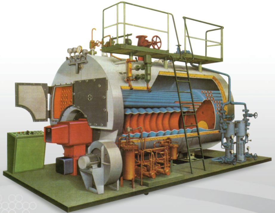
Yatık Buhar Jeneratörü
