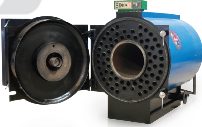
Sıvı/Gaz Yakıtlı Üç Geçişli Sıcak Su Kazanı
