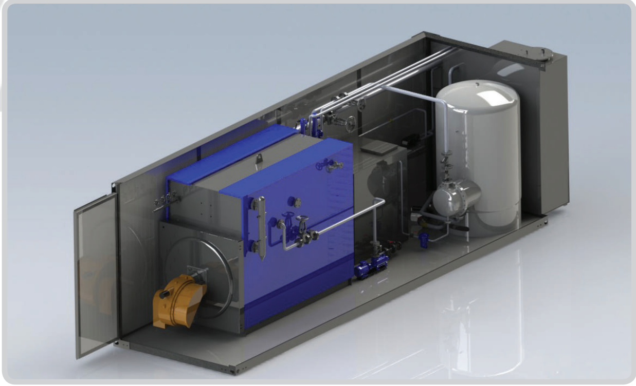
Buhar ve Kullanma Suyu Üreten Mobil Santral
