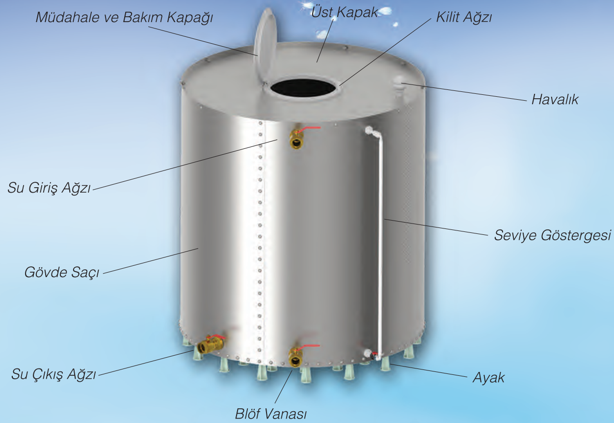
KÜÇÜK KAPASİTE MİNİ MOD SU DEPOSU (MİNİ - MOD)
